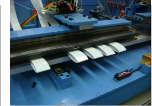
FFCの摺動試験
