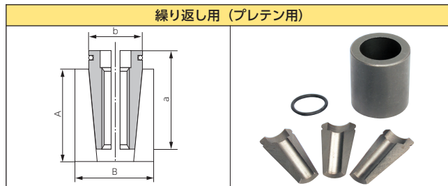
(材質：オスコーン：SCM415H、メスコーン：SCM435H)
