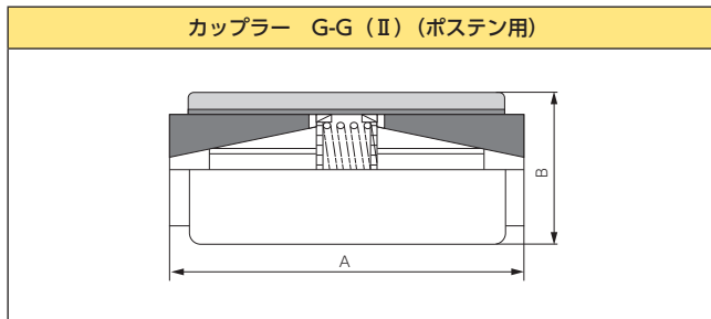
(材質：オスコーン：SCM415H、メスコーン：SCM435H)
