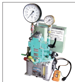
SMP-MINI-N
