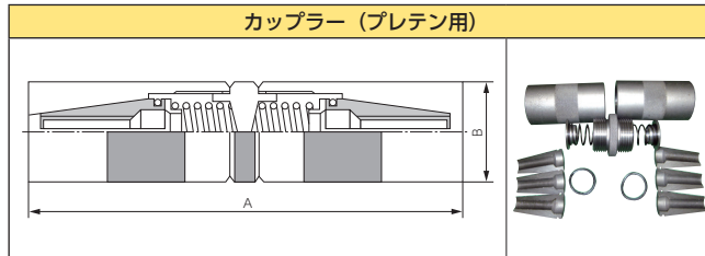
(材質：オスコーン：SCM415H、メスコーン：SCM435H)
