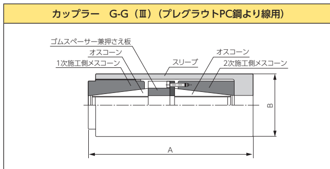
(材質：スリーブ：SCM435H)
