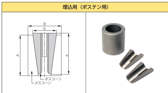
(材質：オスコーン：SCM415H、メスコーン：SCM435H)
