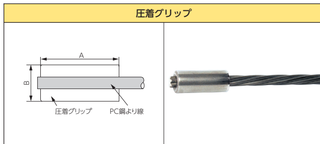
(材質：S55C)
